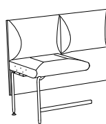
SA810 hörnkoppling (28) H 1030 SH 630 B 1280 D 650
