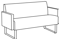
SA620 H 795 SH 450 B 1430 D 630
