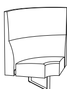
SA640 H 1230 SH 450 B 815 D 815
