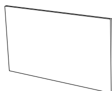
SA350 kupévägg rak (17) H 1315 B 2260 D 45
