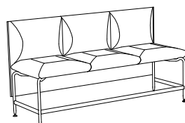
SA830 fristående (15) H 1030 SH 630 B 1910 D 650
