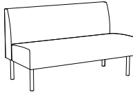
SA620 H 795 SH 450 B 1310 D 630
