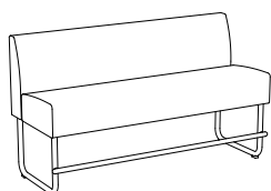
SA630 H 980 SH 630 B 1710 D 640
