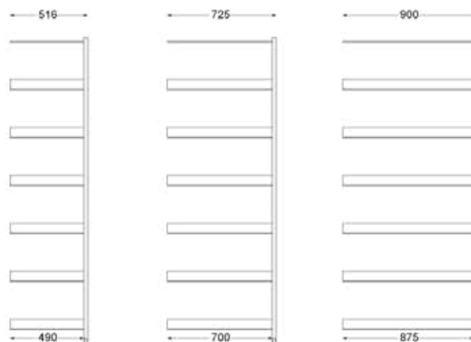
Plussektion
