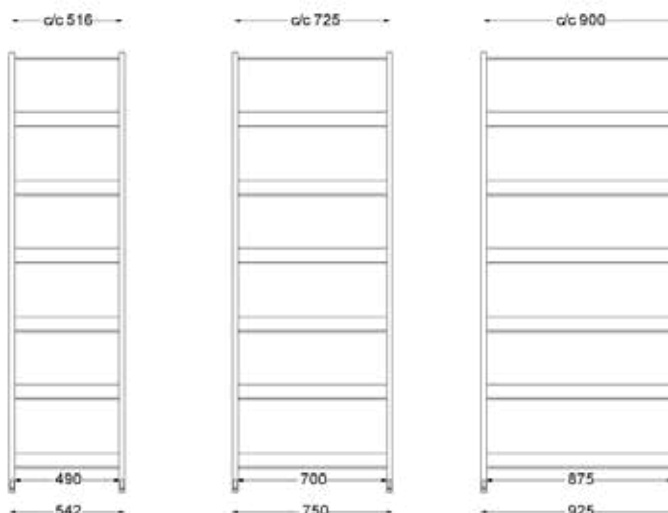
Startsektion
