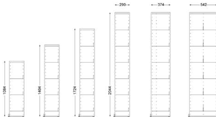
Startsektion
