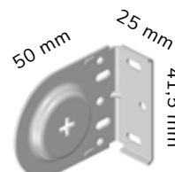
Beslag för takmontage Art.nr. R28157
