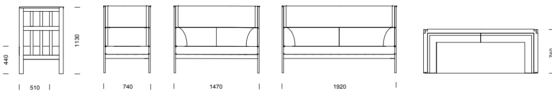
POKER SILENCE ritningar för kombinationer – se sidan 92.
