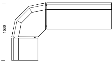
1H3 rundat hörn utan armstöd
