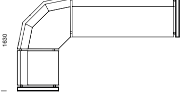
1H3 rundat hörn med armstöd
