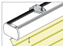
Takmontage, dikt.
