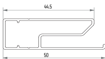
Väggmontering SMALL
