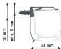
AE-motoriserad AK-kulkedjereglage
