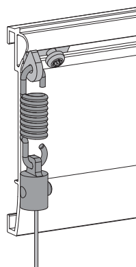
takmontering
