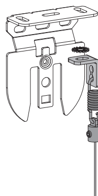
takmontering
