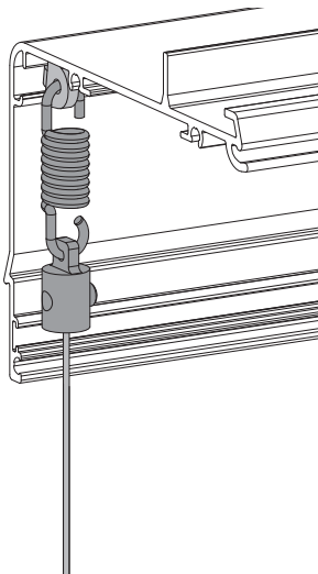
tak/väggmontering
