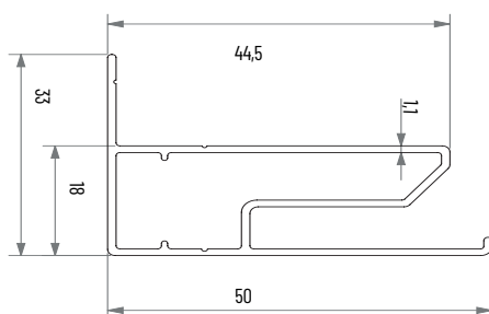
Nischmontering SMALL
