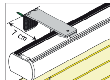
Väggmontage, 70 mm
