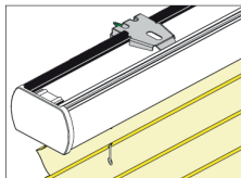
Väggmontage, 5 mm
