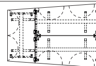
Exempel ihopkoppling av trapetsbord Example of connecting a trapezoidal table
