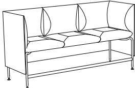
SA830 fristående (13) H 1030 SH 630 B 1940 D 665
