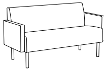
SA620 H 795 SH 450 B 1430 D 630
