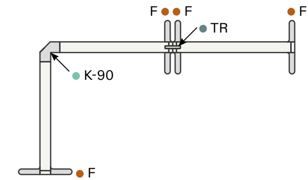
EXEMPEL (Koppling 90°)
