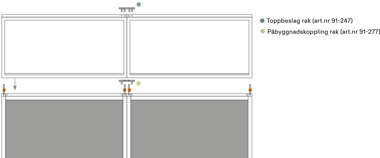
EXEMPEL (Påbyggnadsmodul)
