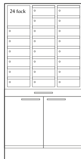
PL9/19 1932 x 910 x 372
