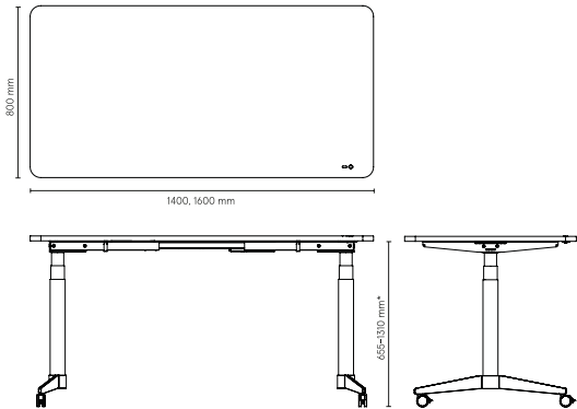
Arbetsbord med hjul och elstativ
