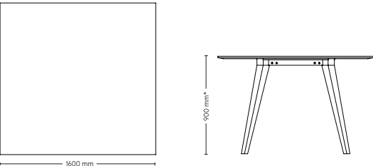
Mötesbord 22: kvadratisk bordsskiva
