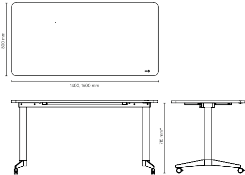
Arbetsbord med hjul och elastativ
