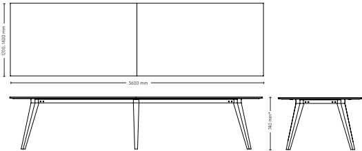
Mötesbord 3: rektangulär bordsskiva
