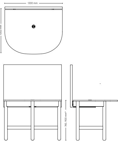
Hybridbord Mini: fast höjd
