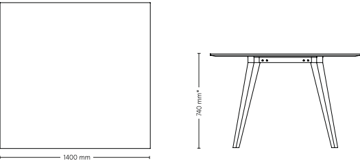
Mötesbord 11: kvadratisk bordsskiva
