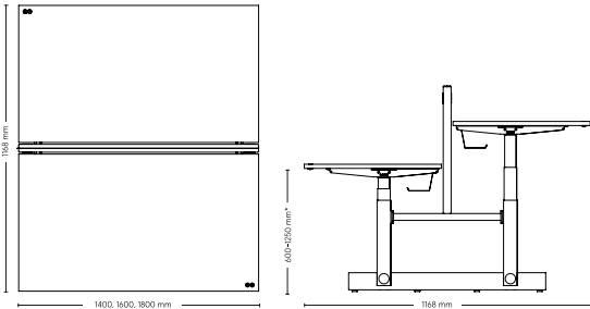
Arbetsbord: 2st med Coinz Twin-fot
