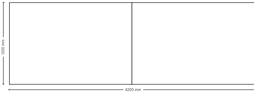
Bordsskiva 4: rektangulär, tvådelad
