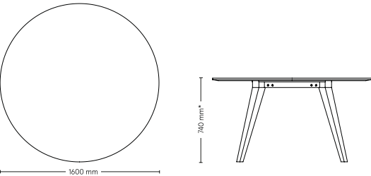
Mötesbord 14: rund bordsskiva
