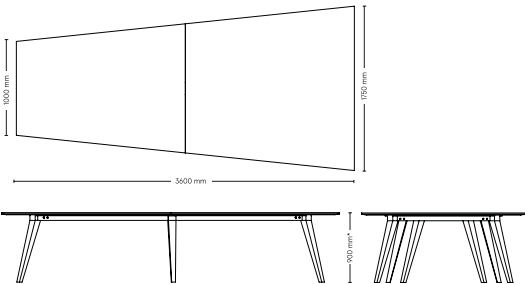
Mötesbord 63: trapetsformad bordsskiva
