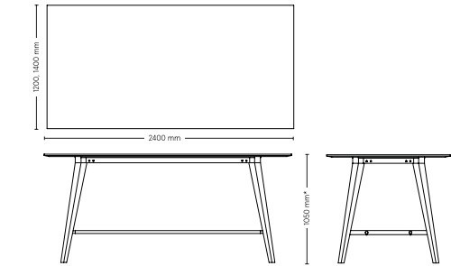
Mötesbord 41: rektangulär bordsskiva
