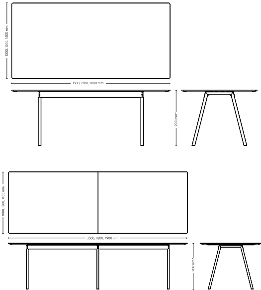
Mötesbord 9: rektangulär bordsskiva
