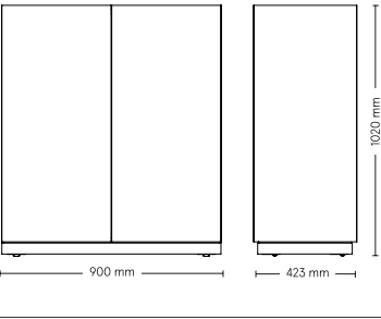
Låg version, dubbelskåp
