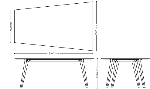
Mötesbord 61: trapetsformad bordsskiva
