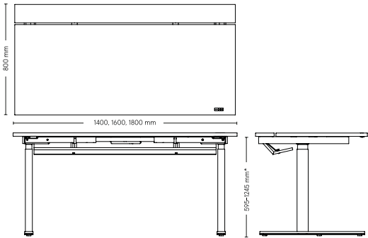
Arbetsbord: delad skjutbar bordsskiva
