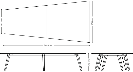
Mötesbord 53: trapetsformad bordsskiva
