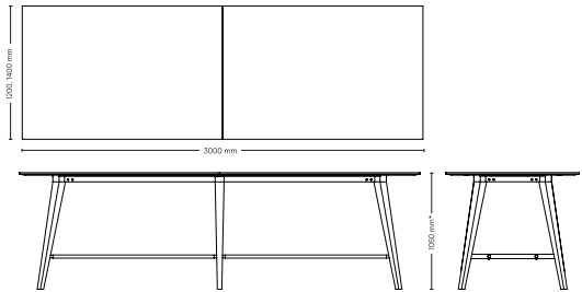
Mötesbord 42: rektangulär bordsskiva
