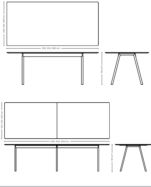
Mötesbord 1: rektangulär bordsskiva
