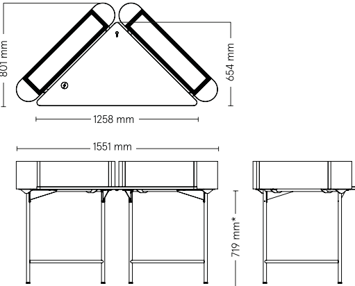
Triangulär bordsskiva - singel
