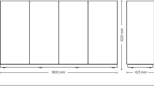
Hög version, enkelskåp
