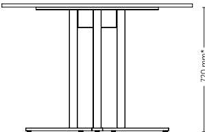
Stativ till bordsskiva 10-13
