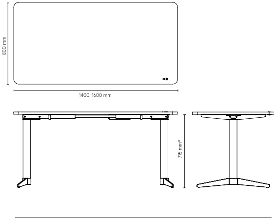
Arbetsbord med ställfot och fast stativ
