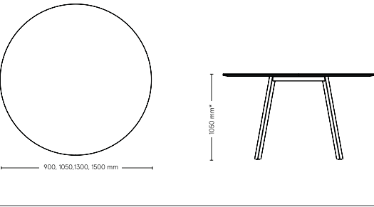
Mötesbord 26, 27, 28: rund bordsskiva
