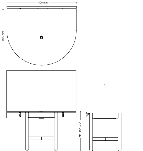
Hybridbord: fast höjd
