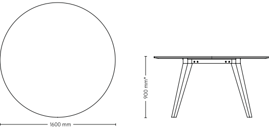
Mötesbord 24: rund bordsskiva
