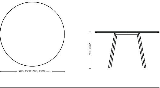
Mötesbord 24, 25: rund bordsskiva
