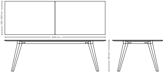
Mötesbord 2: rektangulär bordsskiva
