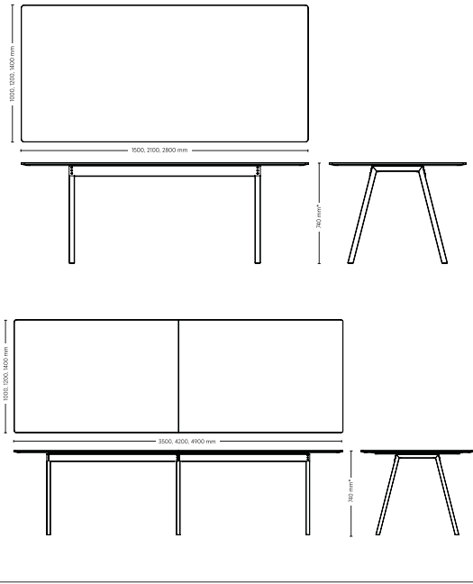
Mötesbord 2: rektangulär bordsskiva
