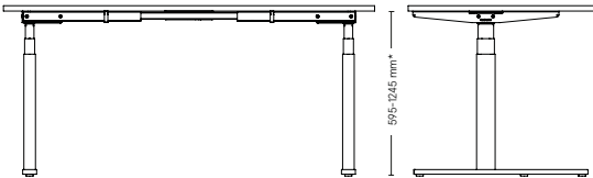
Stativ till bordsskiva 2
