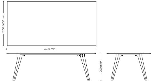
Mötesbord 31: rektangulär bordsskiva
