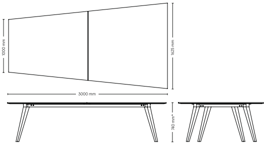
Mötesbord 52: trapetsformad bordsskiva
