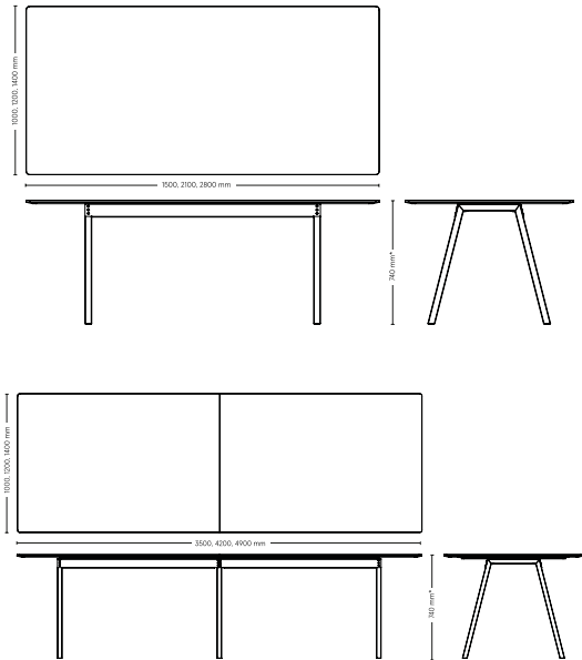
Mötesbord 5: rektangulär bordsskiva
