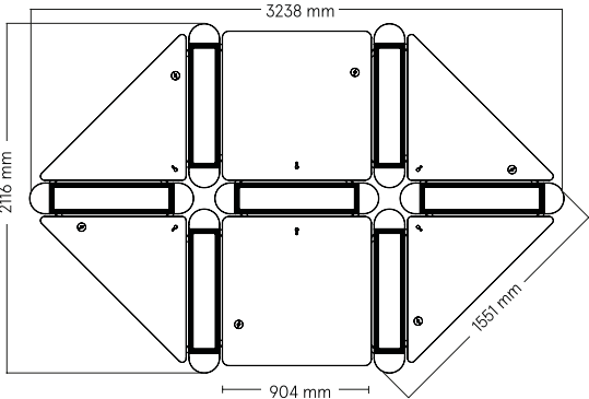
Triangulär-/rektangulär bordsskiva – 4st + 2st i grupp
