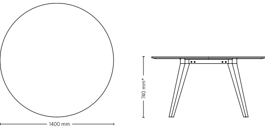
Mötesbord 13: rund bordsskiva
