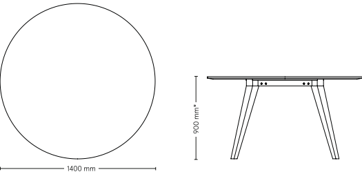
Mötesbord 23: rund bordsskiva
