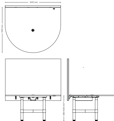
Hybridbord: elektriskt justerbar
