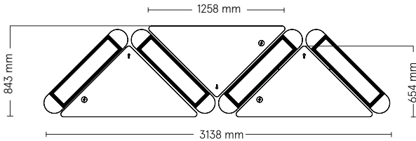
Triangulär bordsskiva - 3st i grupp
