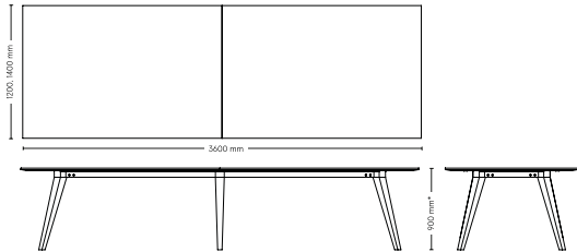
Mötesbord 33: rektangulär bordsskiva
