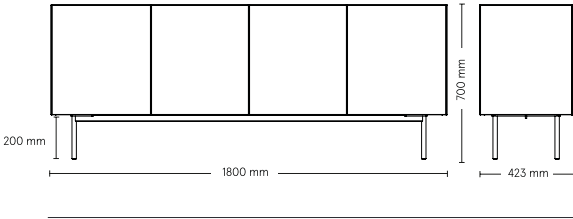
Låg version, dubbelskåp
