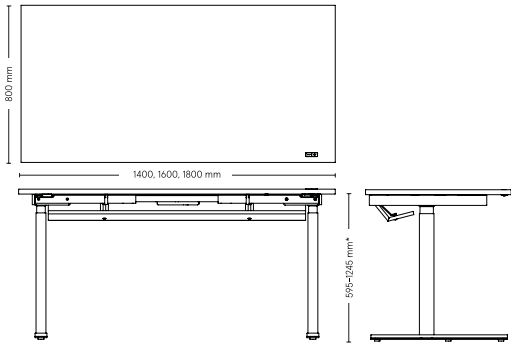
Arbetsbord: fast hel bordsskiva
