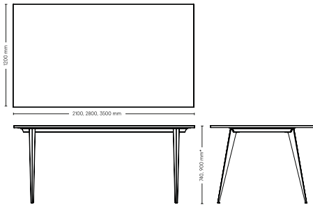
Mötesbord hel skiva
