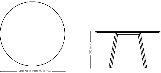
Mötesbord 16, 17: rund bordsskiva
