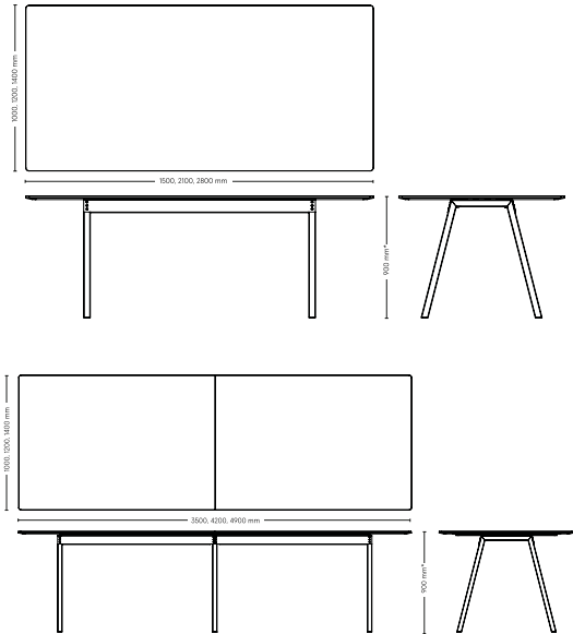
Mötesbord 8: rektangulär bordsskiva
