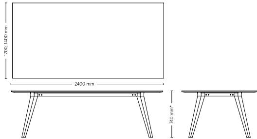
Mötesbord 1: rektangulär bordsskiva
