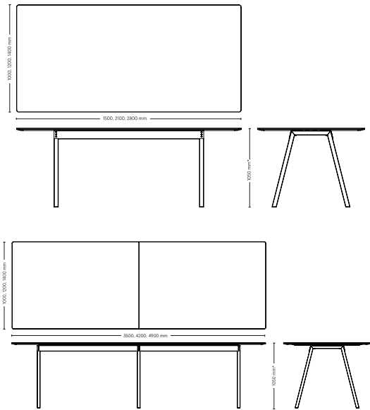
Mötesbord 14: rektangulär bordsskiva
