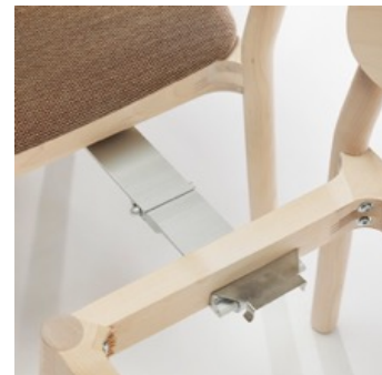
Kopplingsbeslag metall
