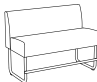
SA620 H 980 SH 630 B 1310 D 640
