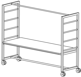
H skiva 730 H 1890 B 2500 D 900
