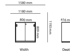
Sliding door
