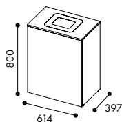
W3312 Hel dörr plats för 60 liters kärl
