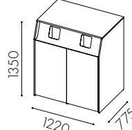
W3521 Hela dörrar för rullkärl 190 liter *
