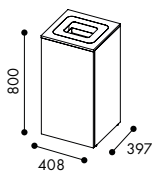
W3311 Hel dörr med säckhållare för 125 liters säck
