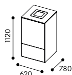
W3212 Dörr ovan till för 1x90 l kärl och lådutdrag undertill *
