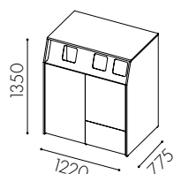
W3523 Hel dörr till vänster för rullkärl 1 l *, dörr ovan till för 2x60 kärl och lådutdrag undertill till höger **
