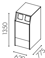
W3520 Dörr ovan till för 2x60 kärl och lådutdrag undertill **
