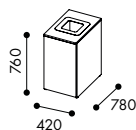
W3217 Låg modul med hel dörr för 1x60 l kärl
