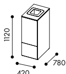
W3214 Dörr ovan till för 1x60 l kärl och lådutdrag undertill **
