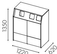
W3516 Dörr ovan till för 90 l kärl i enkelt inkast, 2x60 i dubbelt inkast och lådutdrag undertill **
