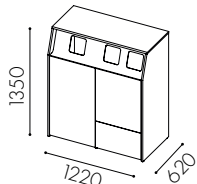
W3515 Hel dörr till vänster för rullkärl 140 l *, dörr ovan till för 2x60 kärl och lådutdrag undertill till höger **
