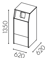
W3511 Dörr ovan till för 90 l kärl och lådutdrag undertill **
