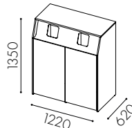
W3513 Hela dörrar för rullkärl 140 liter *
